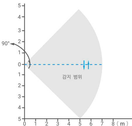
그림 2. 감지 범위의 평면 보기
