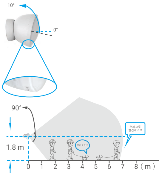
그림 1. 감지 범위의 측면 보기
