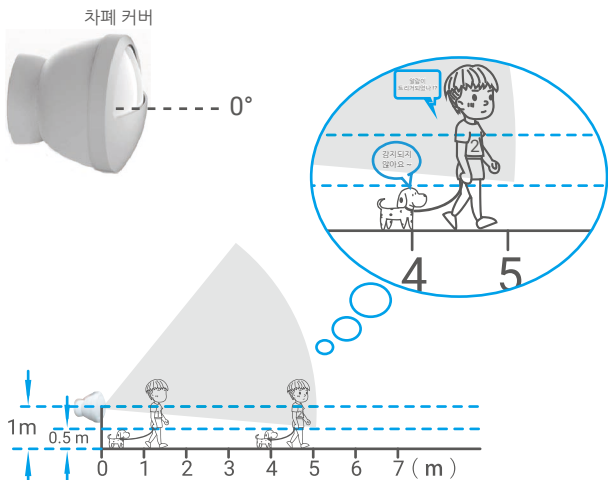
그림 1. 감지 범위의 측면 보기
