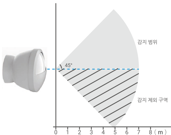
그림 2. 감지 범위의 평면 보기
